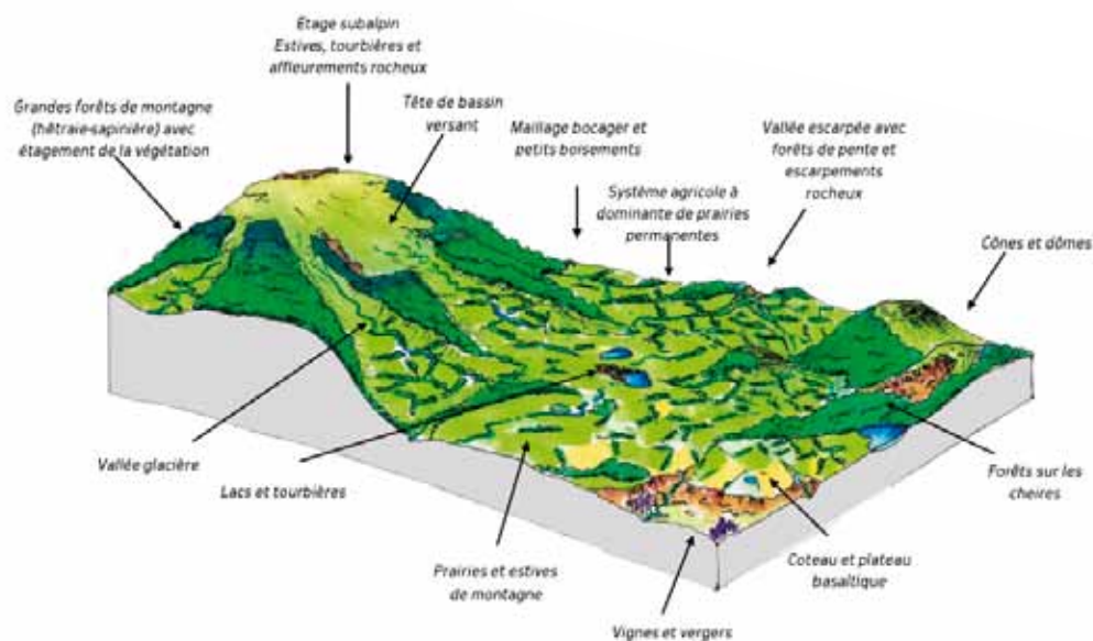
Figure 119 : Bloc diagramme des enchaînements des structures, éléments et motifs écopaysagers de la région naturelle des Volcans d'Auvergne à Corneully
